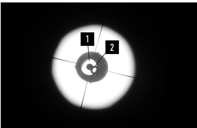
Bild 5. Hauptspiegel dejustiert.
